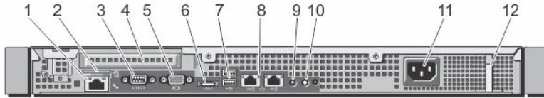
그림 2. 후면 패널 구조 및 표시등
