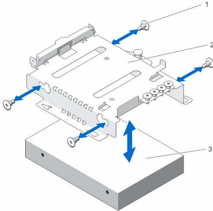
그림 10. 하드 드라이브 케이지에서 3.5인치 하드 드라이브 분리 및 설치
