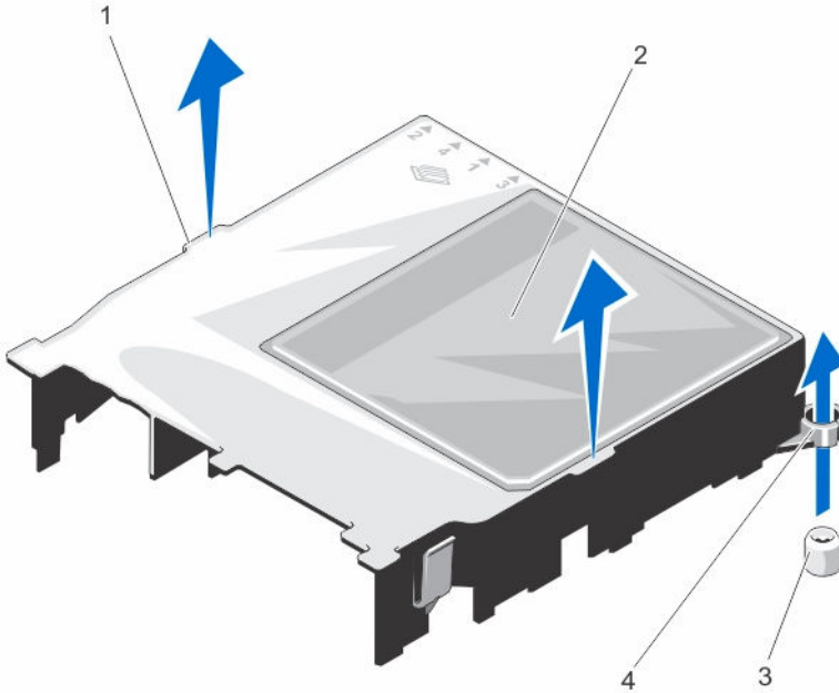
그림 16. 냉각 덮개 분리 및 장착
