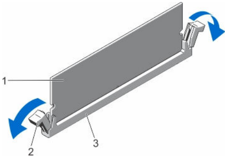
그림 18. 메모리 모듈 분리
