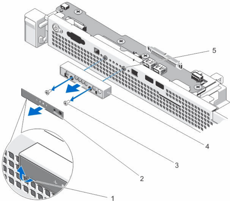
그림 13. LED 모듈 분리 및 설치
