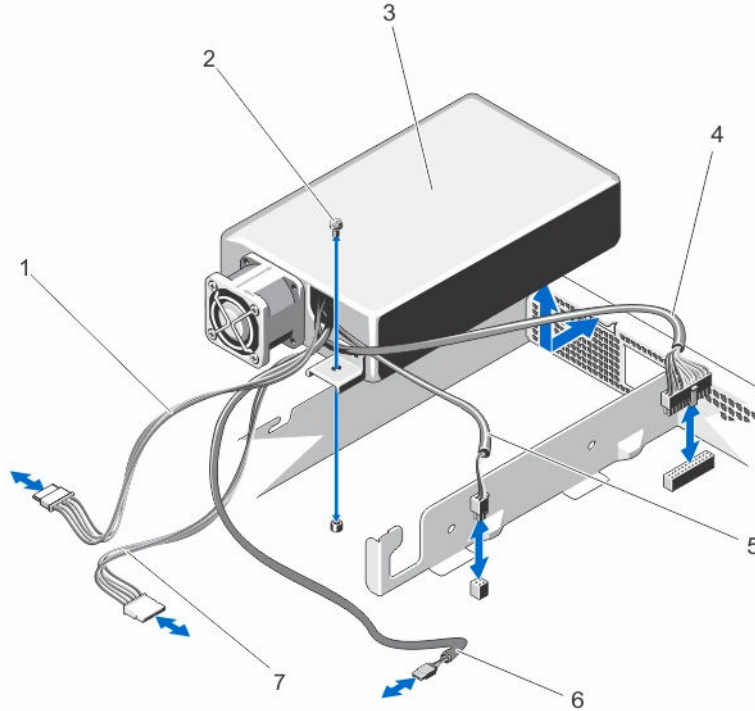
그림 27. 전원 공급 장치 분리 및 설치
