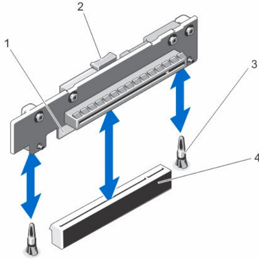
그림 22. 확장 카드 라이저 분리 및 설치
