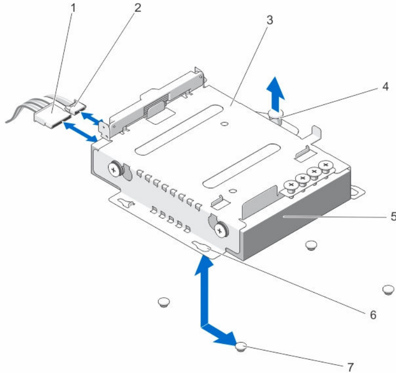
그림 9. 3.5인치 하드 드라이브(HDD1) 케이징 분리 및 설치
