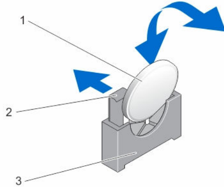
그림 24. 시스템 배터리 장착
