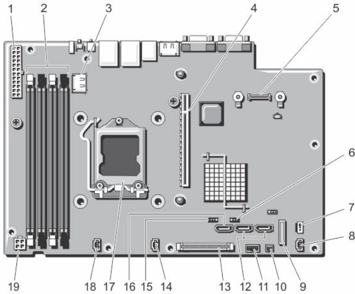
그림 29. 시스템 보드 점퍼 및 커넥터
