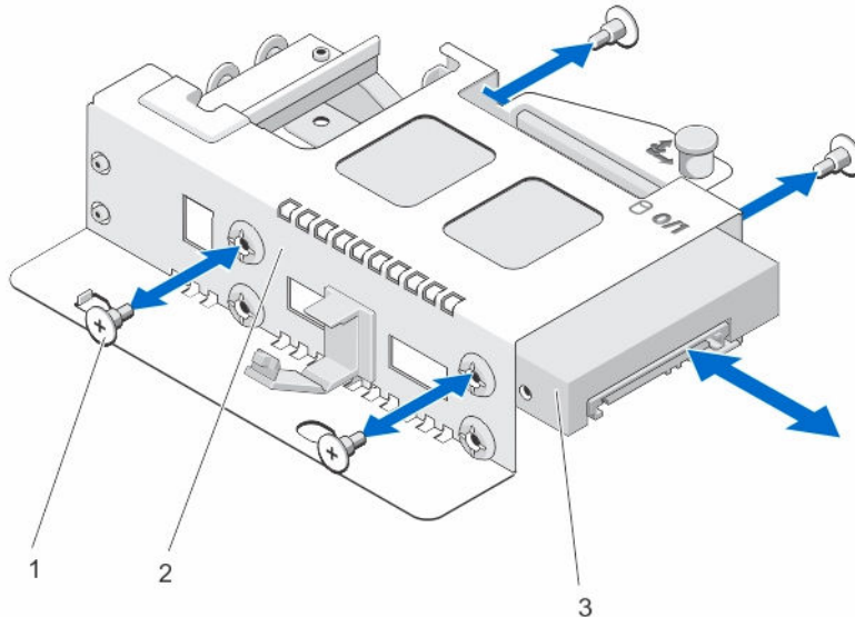
그림 12. 하드 드라이브 케이스에서 2.5인치 하드 드라이브 분리 및 설치
