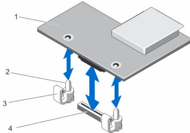
그림 23. iDRAC7 엔터프라이즈 카드 분리 및 설치
