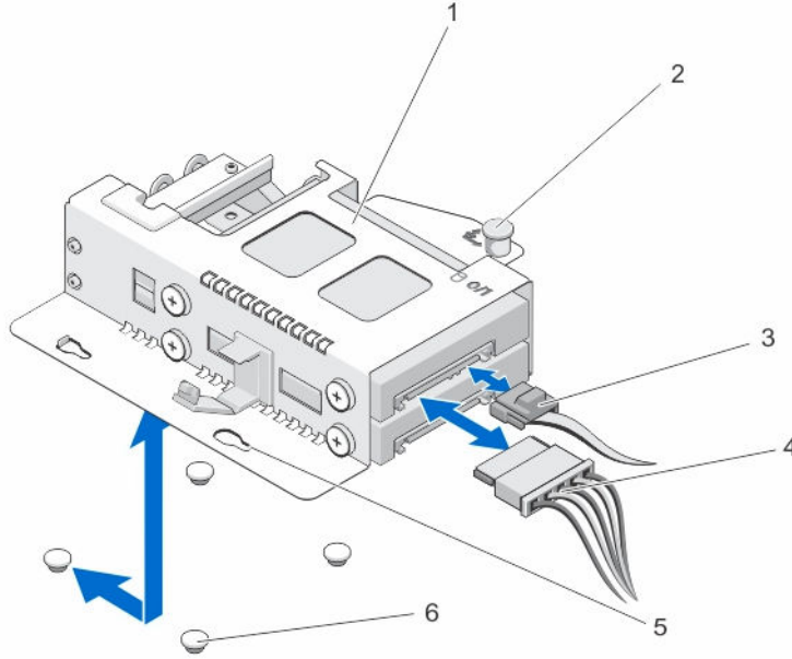
그림 11. 2.5인치 하드 드라이브 케이스 분리 및 설치
