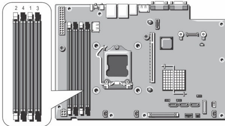
그림 17. 메모리 소켓 위치
