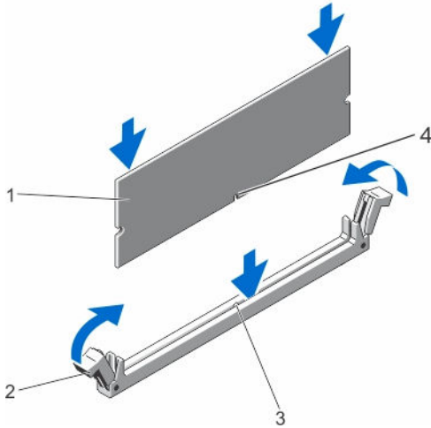
그림 19. 메모리 모듈 설치
