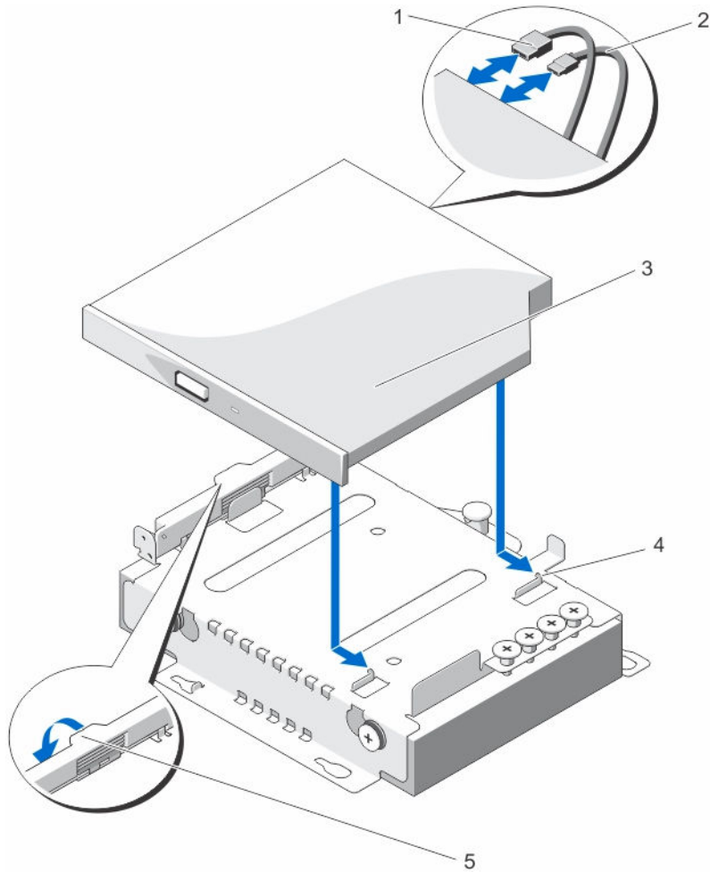
그림 8. 광학 드라이브 분리 및 설치
